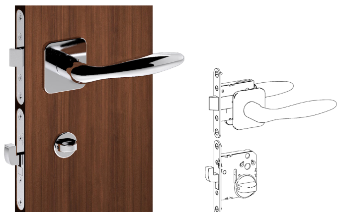
3. Separate lock case (turn knob + key)
